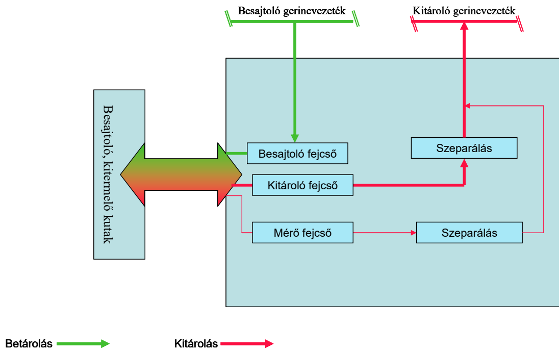
2.sz. ábra Szőreg- 1 gyűjtő- elosztó központok egyszerűsített bloksémája
