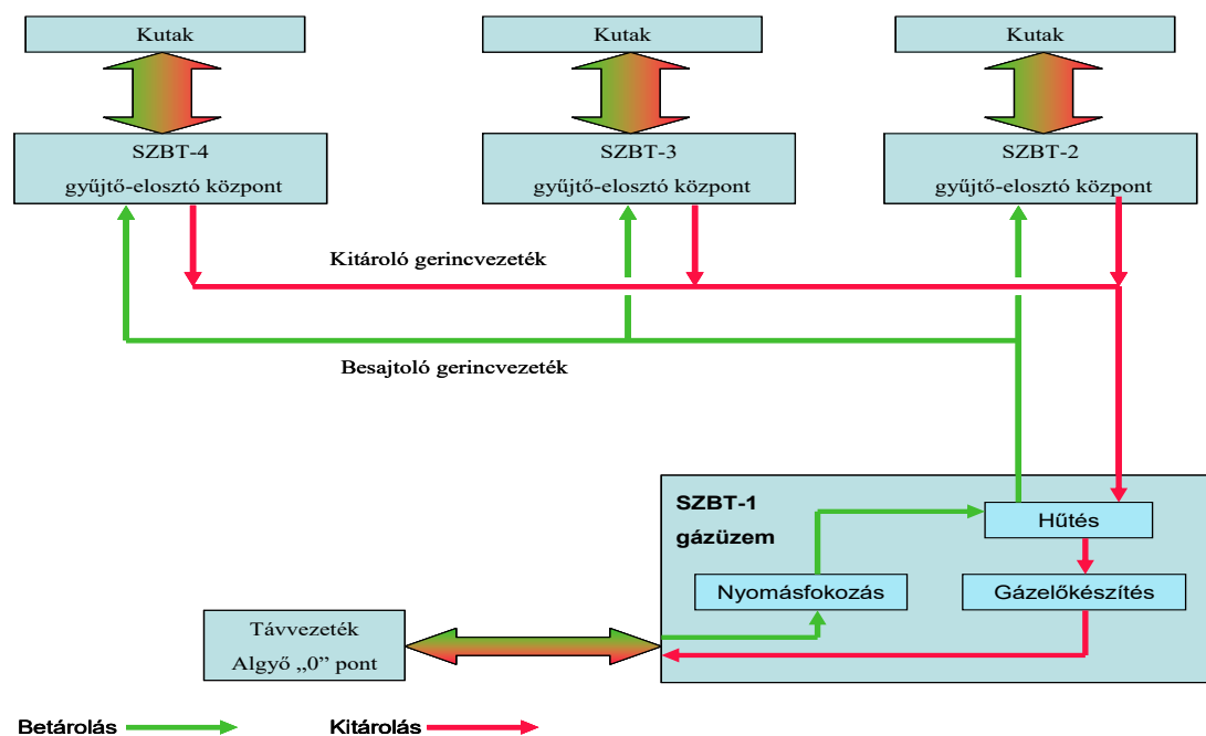
1.sz. ábra Szőreg- 1 tároló technológiai összefüggési bloksémája
