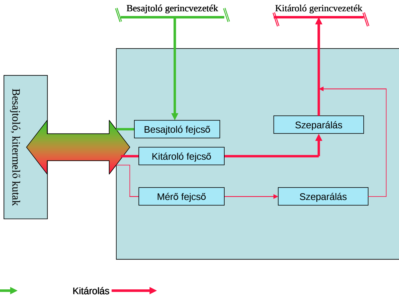
2. sz. ábra Szőreg- 1 gyűjtő- elosztó központok egyszerűsített blokksémája
