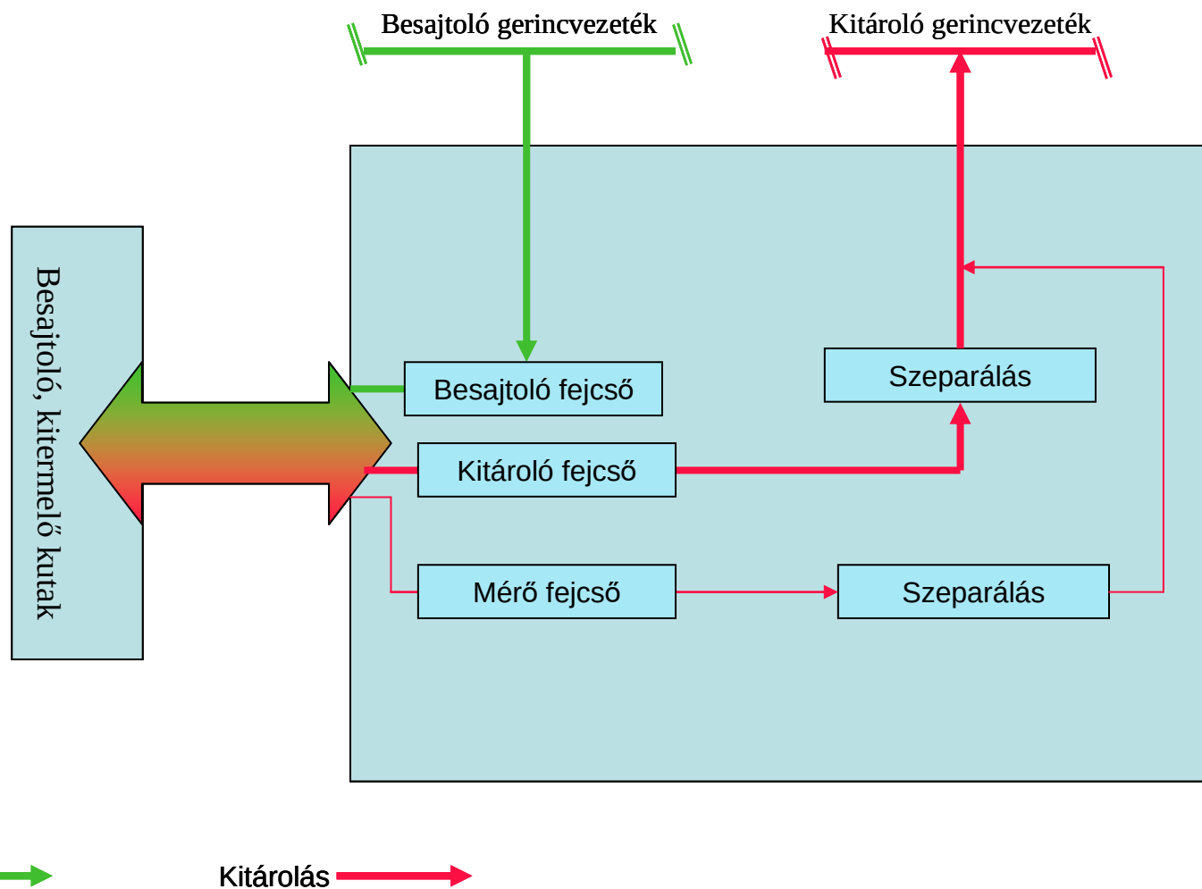
2. sz. ábra Szőreg- 1 gyűjtő- elosztó központok egyszerűsített blokkkép
