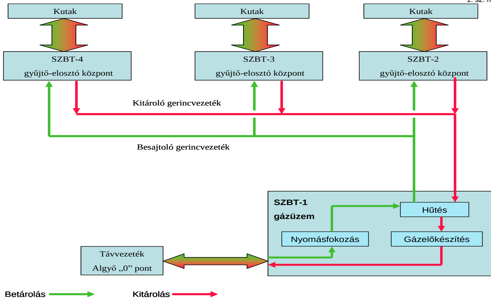
1. sz. ábra Szőreg- 1 tároló technológiai összefüggési bloksémája
