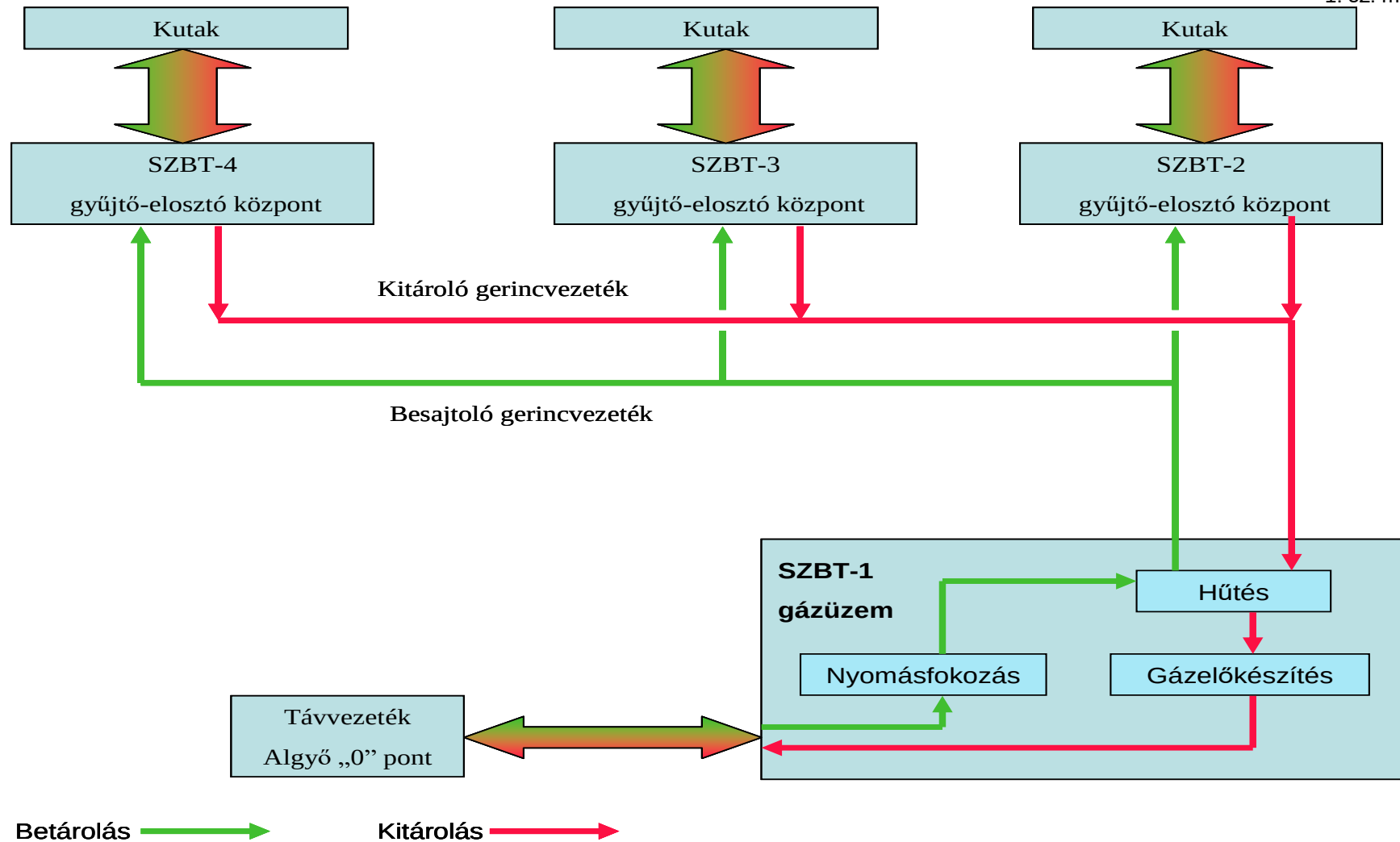
1. sz. ábra Szőreg- 1 tároló technológiai összefüggési bloksémája
