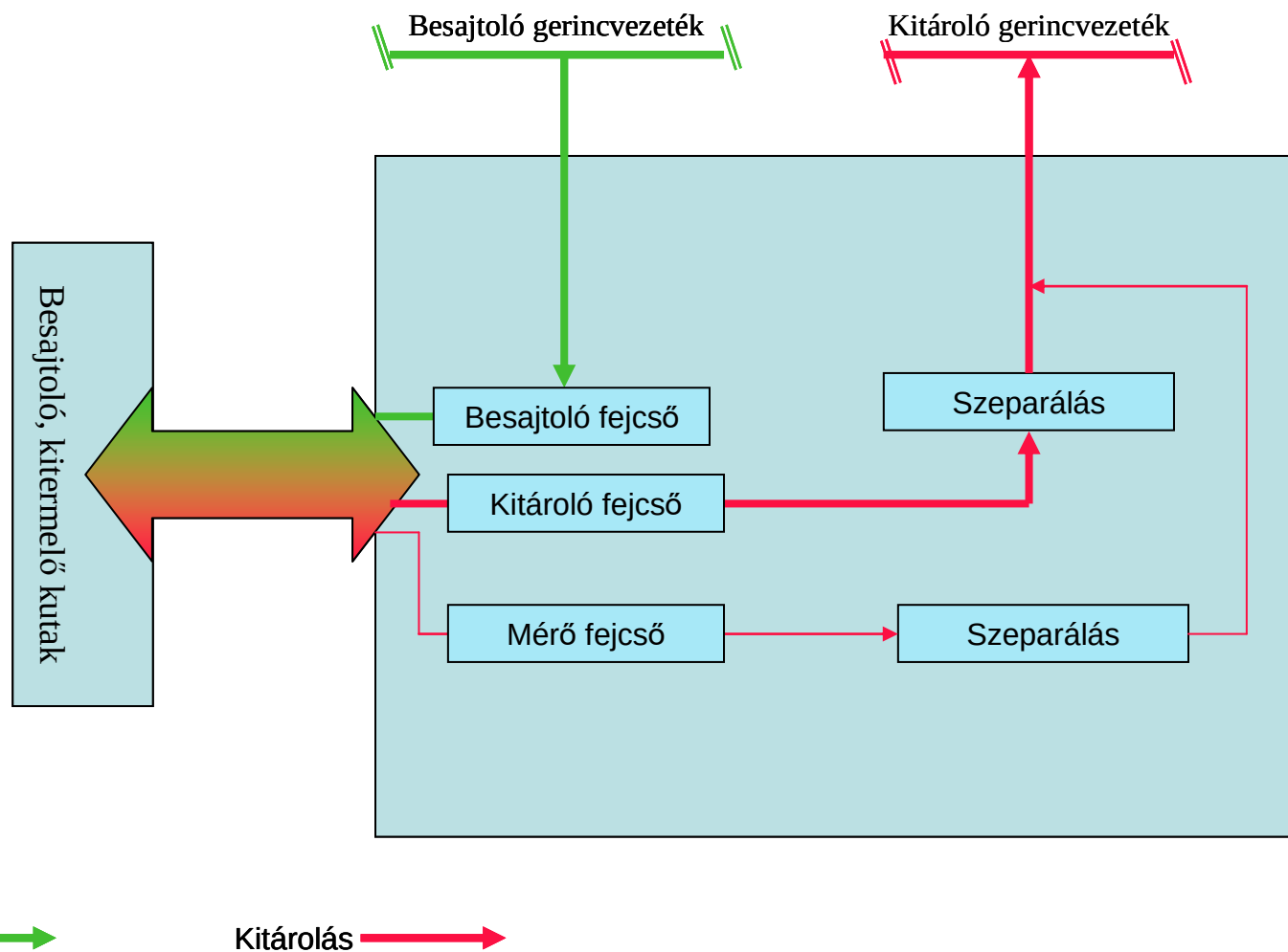
2. sz. ábra Szőreg- 1 gyűjtő- elosztó központok egyszerűsített bloksémája
